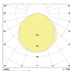
Lichtverteilungskurve IndustryLUX long ultra 1200
