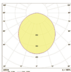
Lichtverteilungskurve IndustryLUX long 1200
