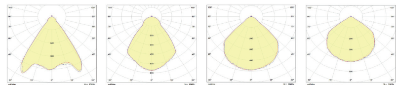
Lichtverteilungskurve IndustryLUX 110 IP40
