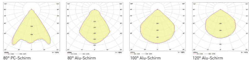
Lichtverteilungskurve IndustryLUX 110 IP65
