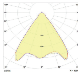
Lichtverteilungskurve IndustryLUX 068 IP65
