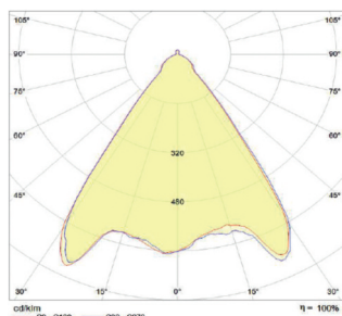
Lichtverteilungskurve IndustryLUX 068 IP40
